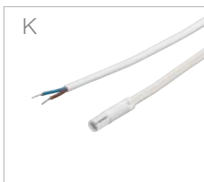
K Anslutningskabel för anslutning mellan transformator och Mini Plug-system. 230V/2,5A
